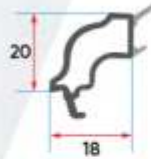
ER 6008 Dekoratif Çift Cam Çıtası Decorative Double Glazing Bead
