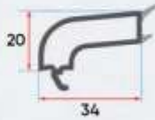
ER 6026 Oval Tek Cam Çıtası Ovoid Single Glazing Bead
