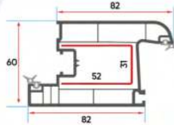
ER 6025 Oval Kapı Kanat Profili Ovoid Door Sash Profile
