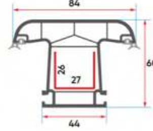
ER 6023 Oval Orta Kayıt Profili Ovoid Mullion Profile
