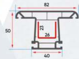
S 1034 Sürme Orta Kayıt Sliding Mullion
