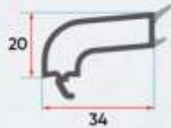
ER 6026 Oval Tek Cam Çıtası Ovoid Single Glazing Bead
