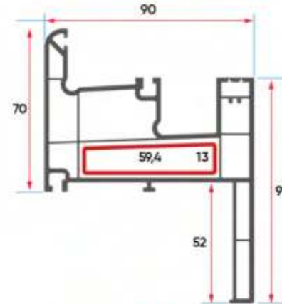
S 1031 Sürme Tekli Pervazlı Kasa Sliding Single Frame with Cornice
