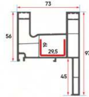
S 1026 Sürme Pervazlı Çiftli Kasa Sliding Double Frame with Cornice
