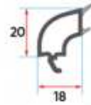
ER 6027 Oval Çift Cam Çıtası Ovoid Double Glazing Bead
